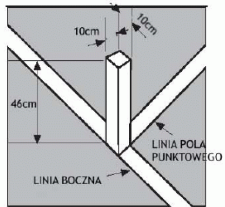
WYMIARY PYŁONU (SŁUPKA WYZNACZAJĄCA ROGI POLA PUNKTOWEGO)
