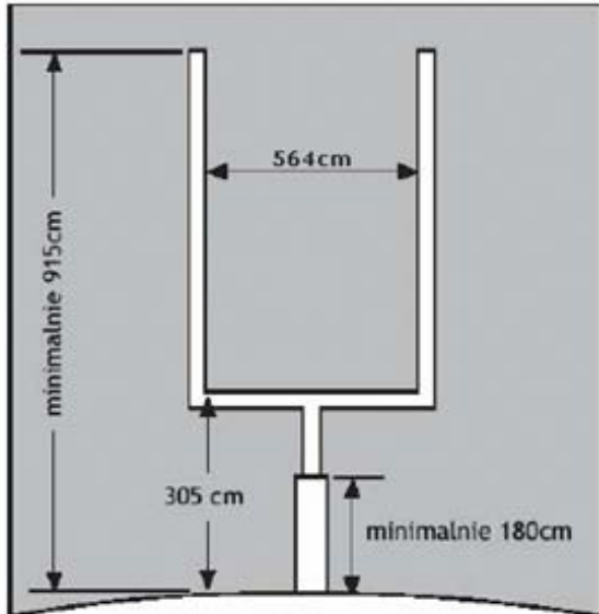
WYMIARY BRAMKI
